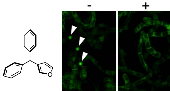
図 2. chem7 の構造（左）とタバコ培養細胞を用いた細胞分裂活性の判定（右）
