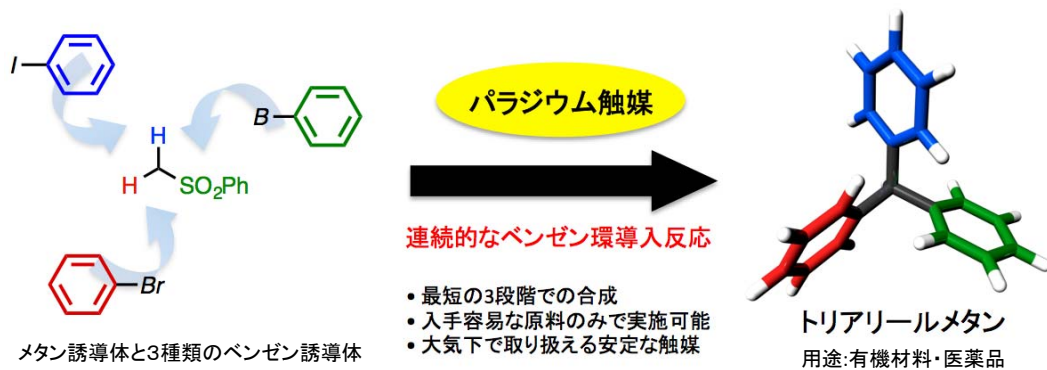
図 1. パラジウム触媒を用いたトリアリールメタンの最短工程合成
