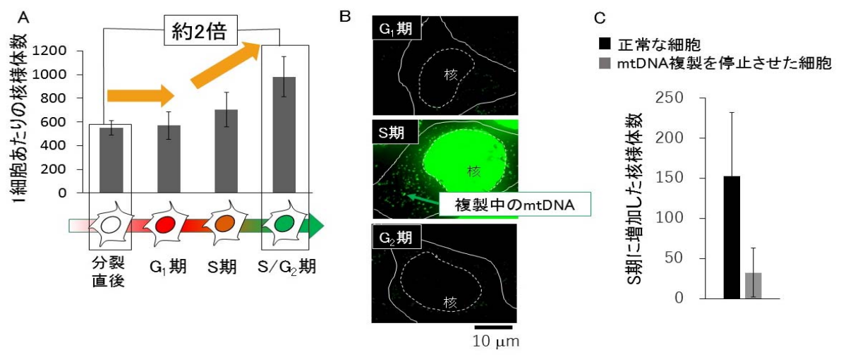
図 3. 細胞周期におけるミトコンドリア様体数と mtDNA 複製の制御 (A)細胞周期の様々な時期の核様体数 (B)細胞周期における mtDNA 複製の様子 (C) mtDNA 複製を停止させたときの核様体数の変化
