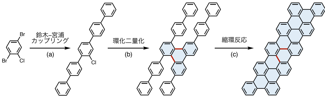
図5 ナノグラフェンの3ステップ合成
