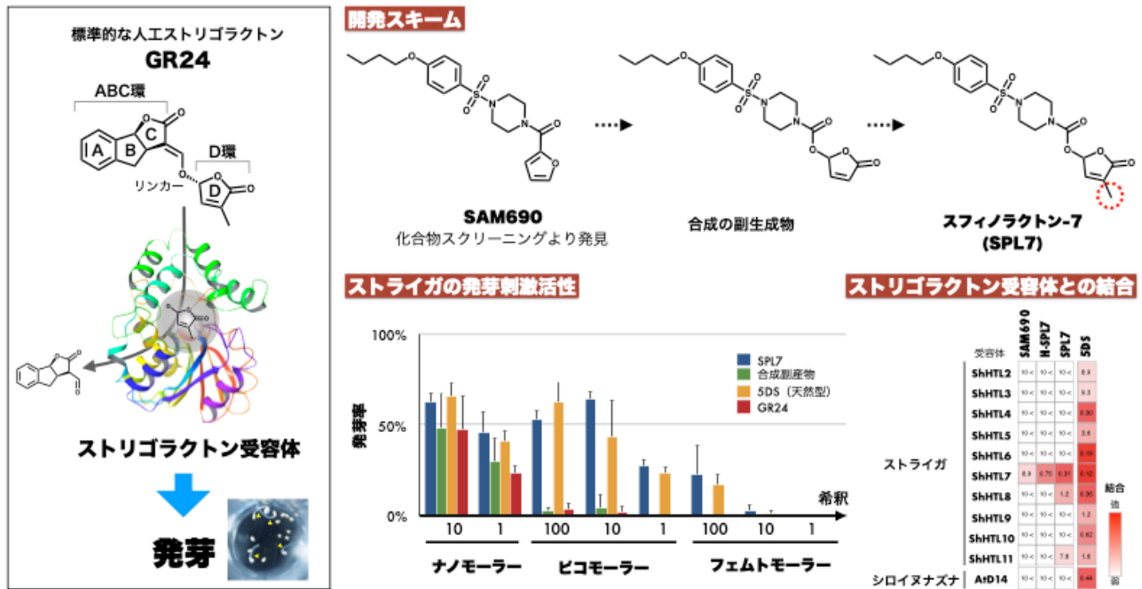
図3: ストライガに選択的に作用する人工ストリゴラクトンの開発。(左)ストリゴラクトンの D 環部位は、受容体と直接つながる特に重要な部位であるが、ABC 環の構造はフレキシブルに改変できる。(右)そこで、12,000 化合物ライブラリーより、ストライガの受容体だけに作用する化合物の選抜を行なったが、その過程で見つかった化合物合成の副生成物は、D 環とよく似た構造をもつ非常に活性の高いハイブリット分子であることが明らかとなった。最適化した分子「スフィンラクトン 7 (SPL7)」は、非常に低濃度であるフェムトモラー (1/10 13-15 mol/L) の範囲でもストライガの発芽を誘導する非常に高い活性をもっているにも関わらず、ストライガのストリゴラクトン受容体 ShHTL7 に対する選択性が高く、モデル植物であるシロイヌナズナ の受容体 AtD14 には結合しない分子であることが判明した。
