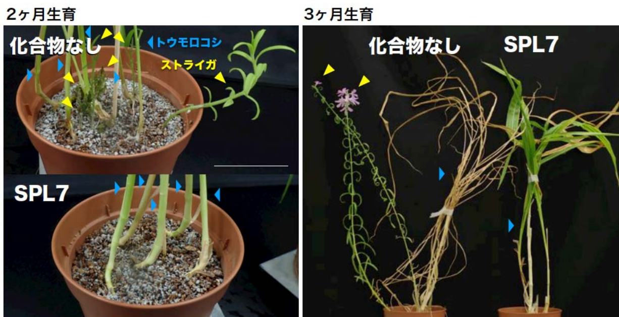
図4: SPL7を用いた自殺発芽試験。SPL7で土を前処理し、自殺発芽を誘導することで、ストライガのトウモロコシへの寄生を抑えることができた。
