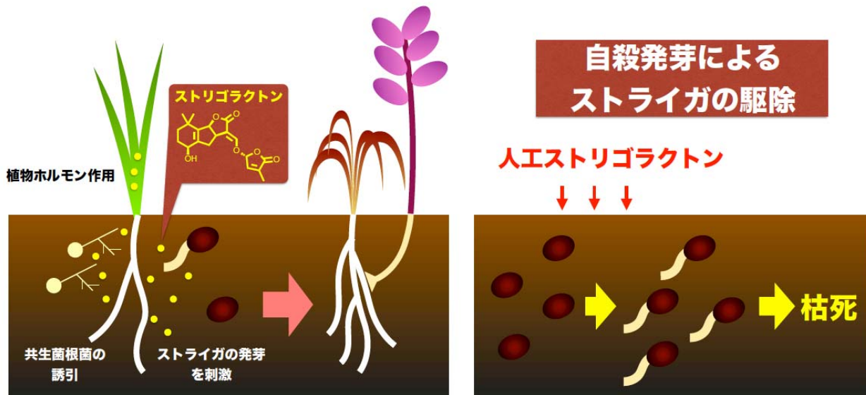
図 2: 自殺発芽によるストライガの駆除法。(左)休眠しているストライガ種子は、宿主の根から土中に放出されるストリゴラクトンに反応して発芽する。ストリゴラクトンは、本来、共生する菌根菌を根に呼び寄せるシグナルである。また、植物ホルモンとして枝分かれの抑制や根毛の成長に関わる。(右)ストライガの種子は宿主がいないところで発芽してしまうと 4 日程度で死んでしまう。そこで、人工ストリゴラクトンを用いて作物のないところで強制的にストライガの種子を発芽させる「自殺発芽」によってストライガの種子を土壌から除くことができる。この方法を実践するには、ストライガだけに作用する強力な人工ストリゴラクトンの開発が必須である。
