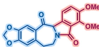
デオキシチレニン 天然有機化合物
