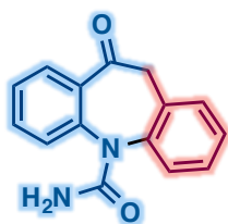
オキシカルバゼピン 抗てんかん薬
