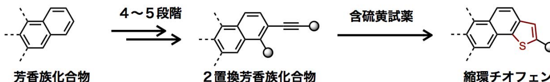
図2 チオフエン縮環反応の従来法
