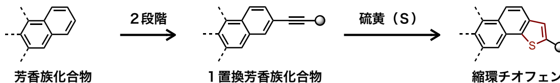
図3 今回開発したチオフエン縮環反応
