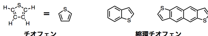
図1 チオフエンと縮環チオフエンの構造
