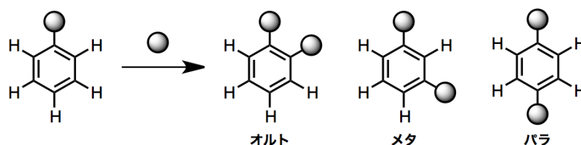
図1 2置換ベンゼン
