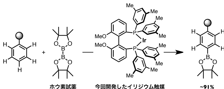
図2 今回開発したイリジウム触媒によるベンゼン環のホウ素化反応
