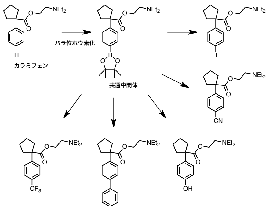
図3 カラミフェンのベンゼン環パラ位ホウ素化を経た2段階誘導化
